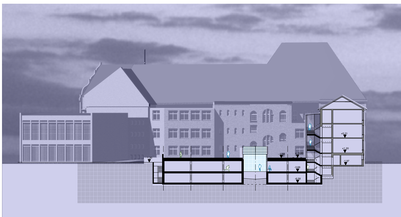
Längsschnitt Innenhof 1:200
