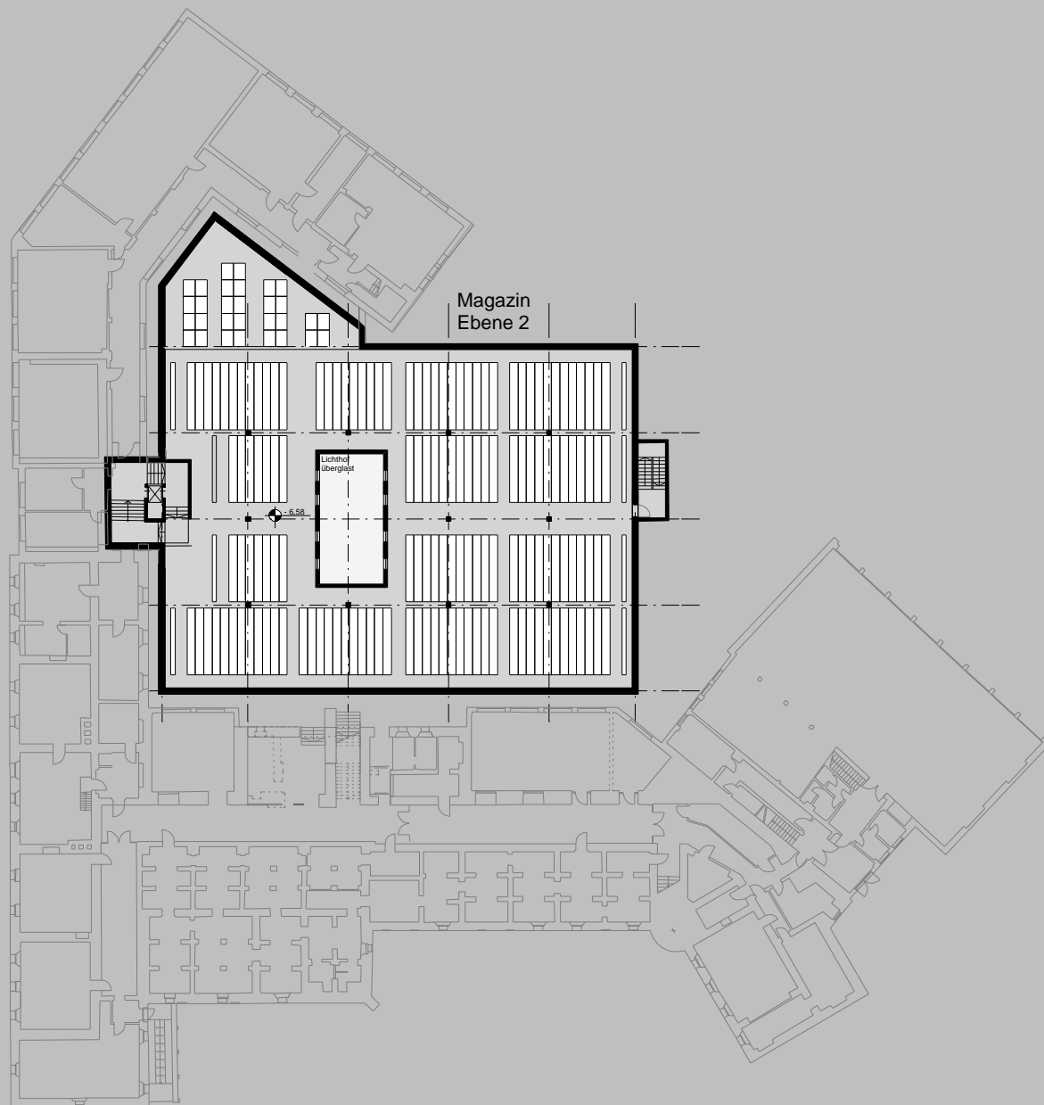
Grundriss Magazinbereich 1:200
