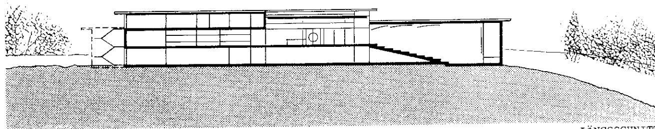
LÄNGSSCHNITT
