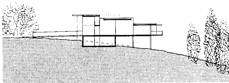
QUERSCHNITT
