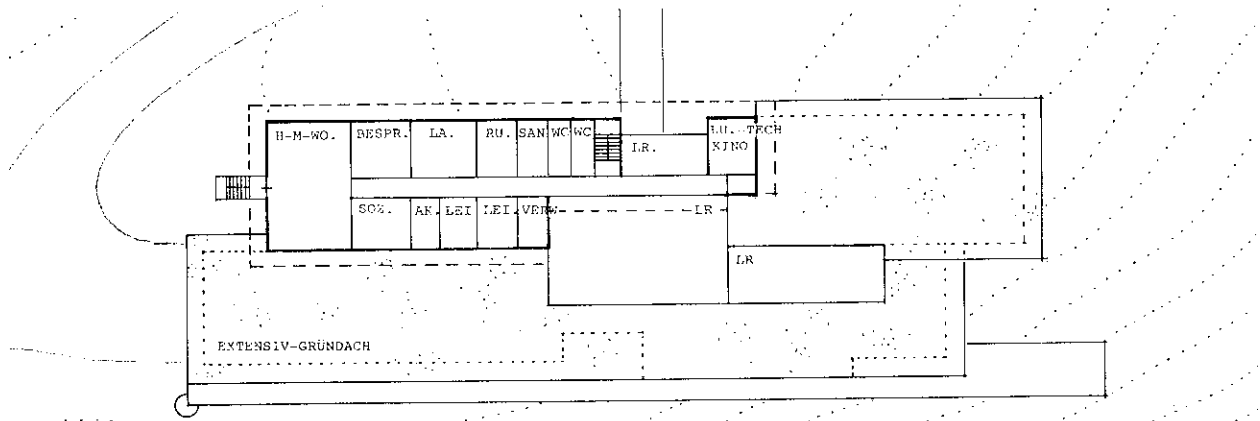
GRUNDRISS OG +685,00
