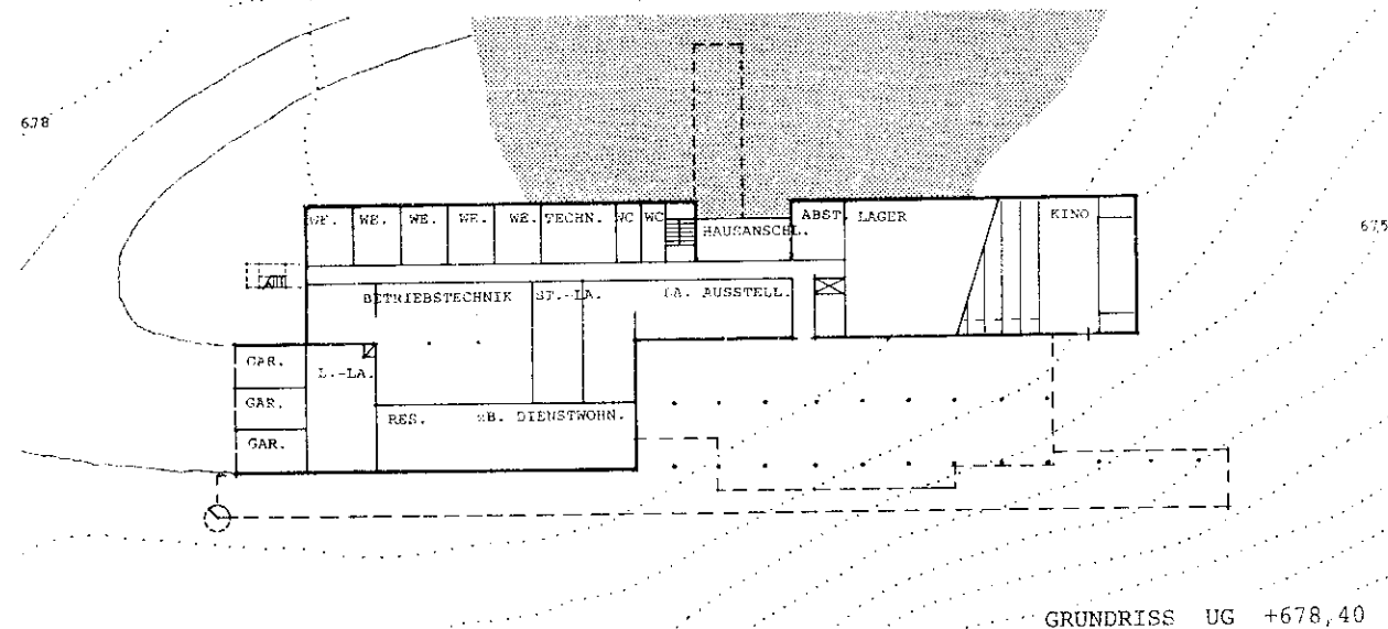
GRUNDRISS EG +681,70
