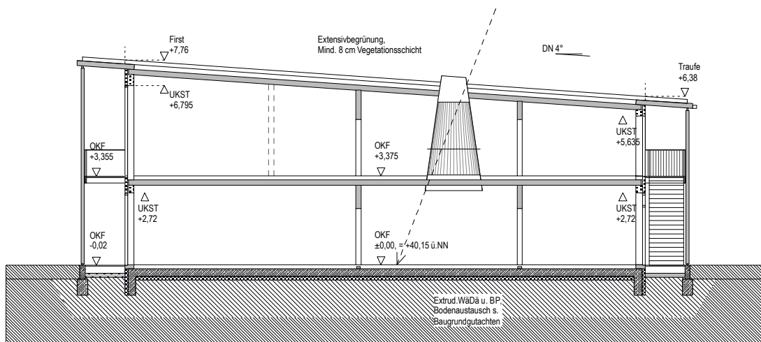
QUERSCHNITT
